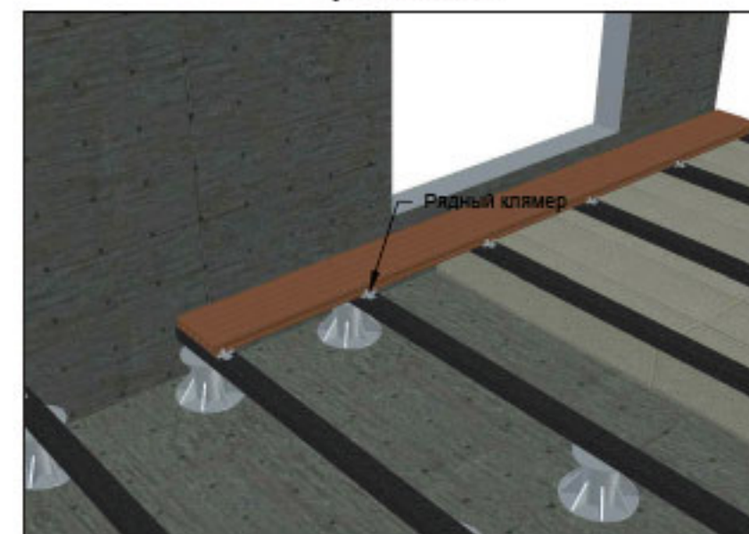
укладка досок
