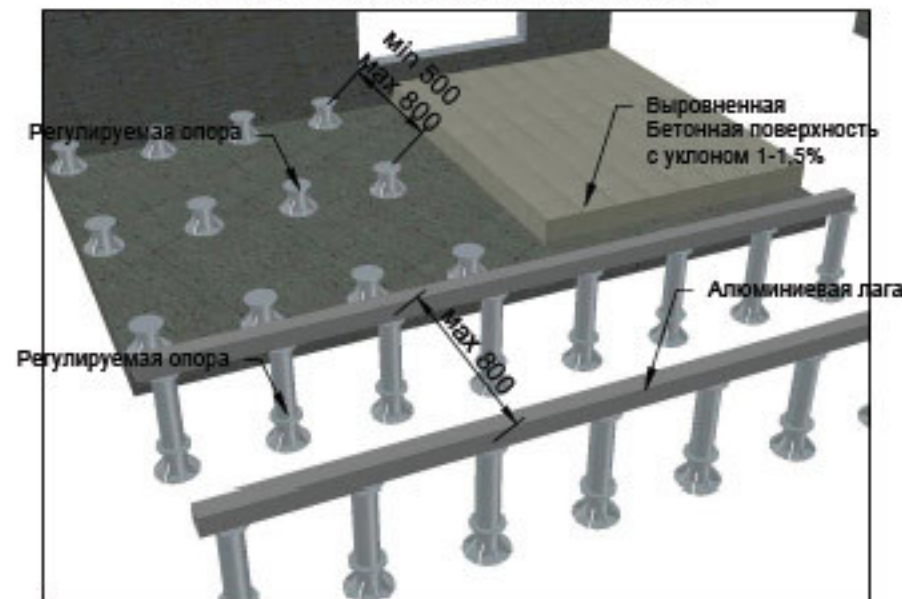
Выравнивание основания для укладки лаг
