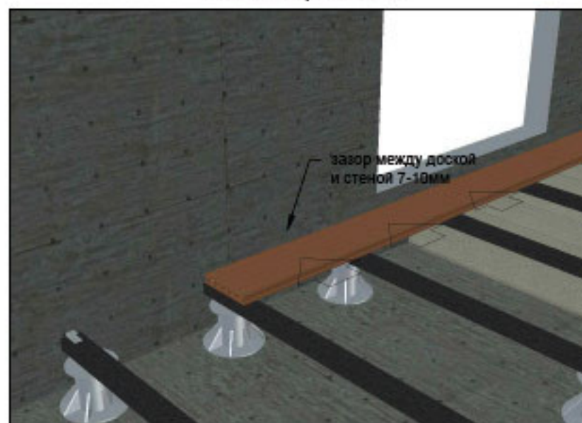
монтаж первой доски
