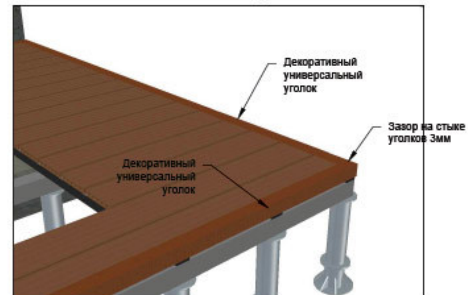
внешняя отделка
