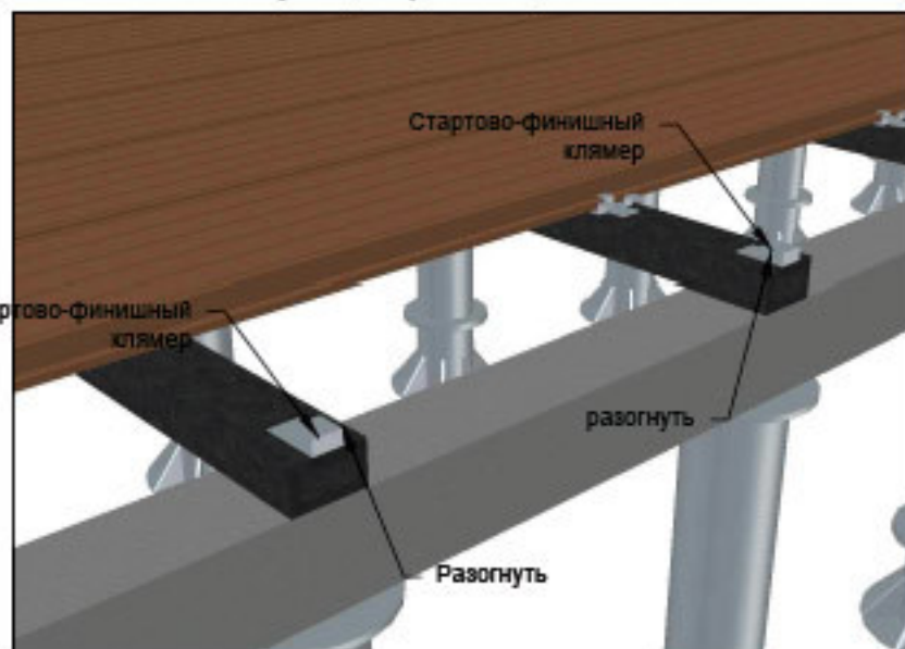
укладка трассной доски
