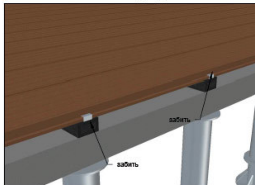
монтаж последней доски
