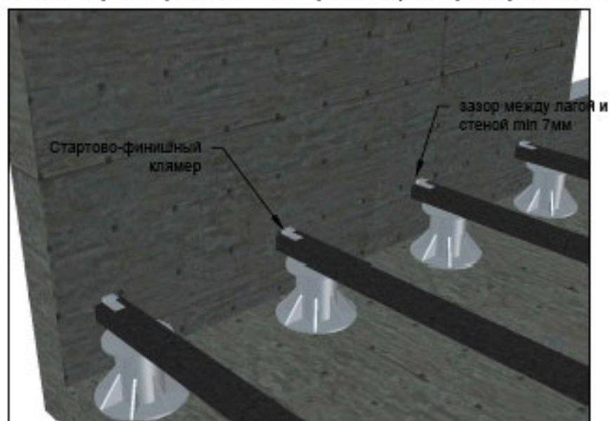
монтаж стартово-финишных клямеров для фиксации первой доски
