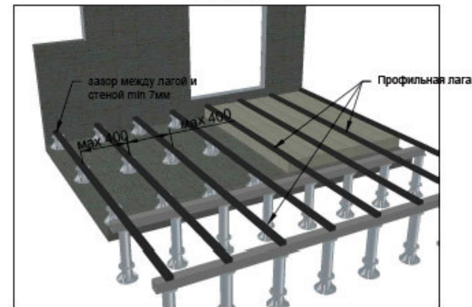
укладка лаг
